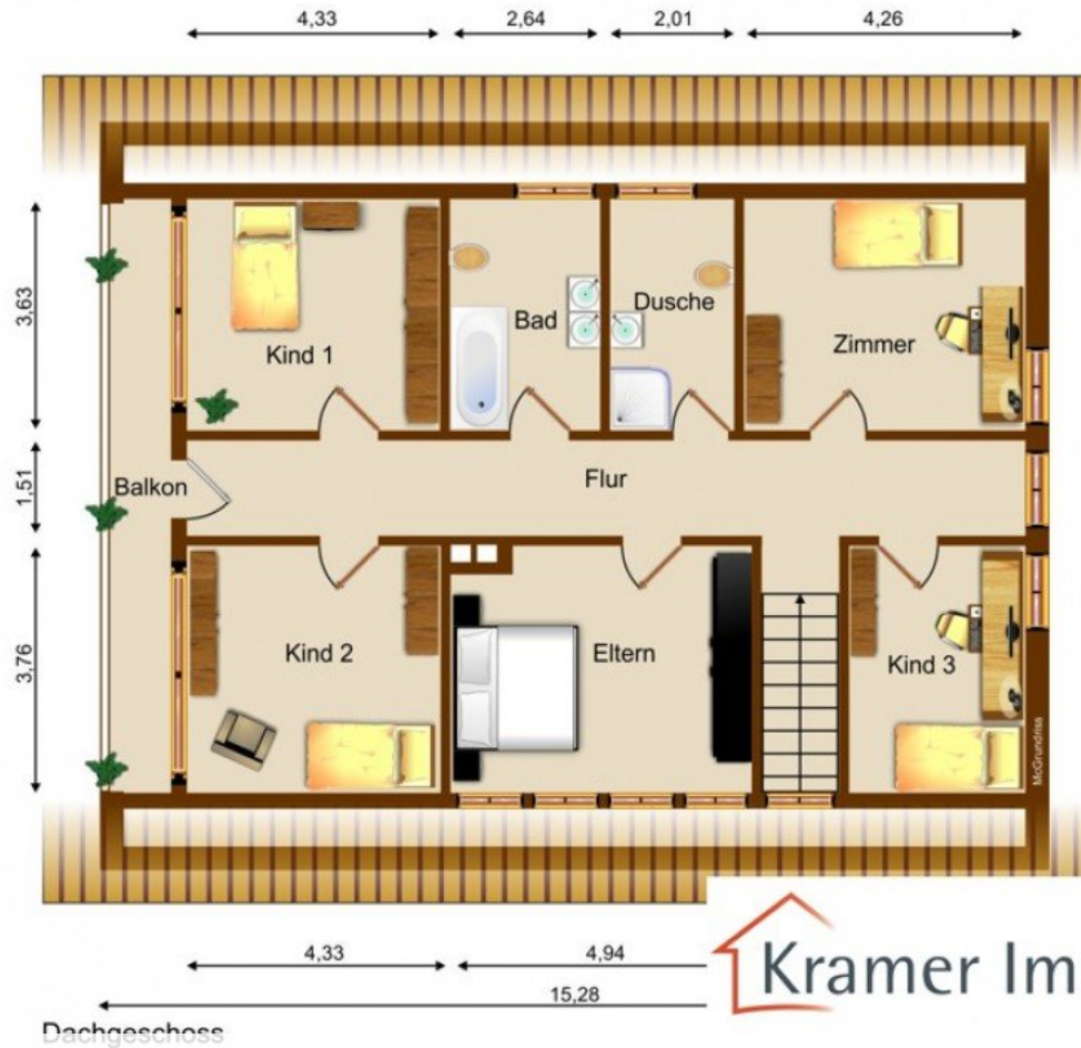
Grundriss Dachgeschoss
