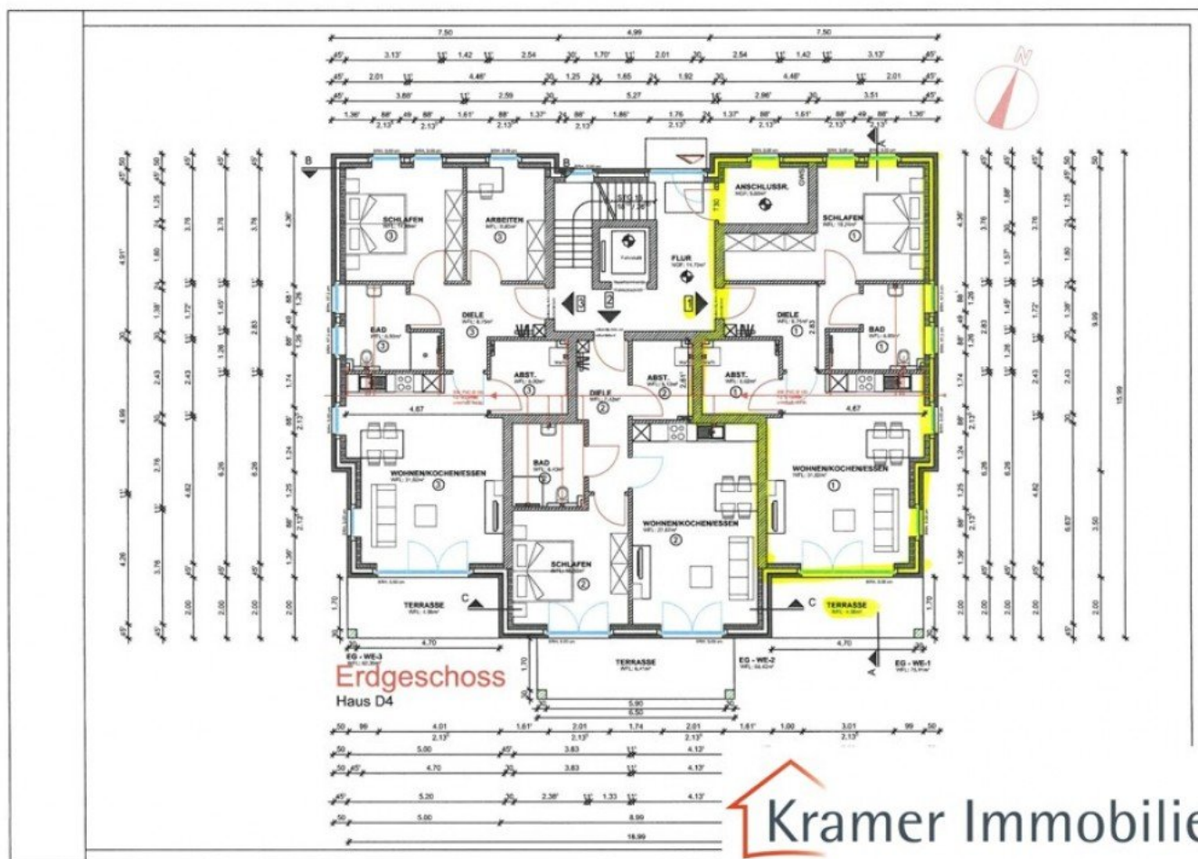
Grundriss EG-Wohnung Nr. 1
